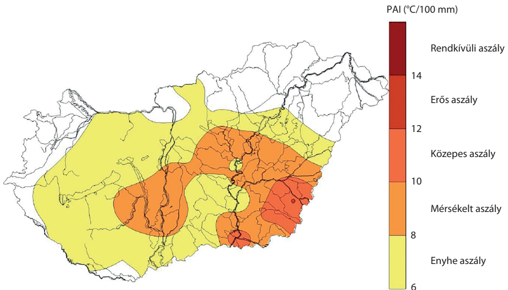
3.36. ábra Az aszályindex (PAI) 2021-re számított értékeinek területi eloszlása
