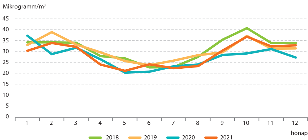
7.2. ábra A nitrogén-dioxid átlagos havi koncentrációja Budapesten
